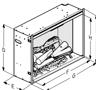
Afmetingen haard
