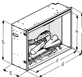
Feuerkammer Dimensionen
